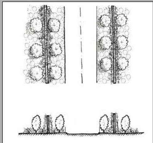
2 mitigazione di barriera antirumore
