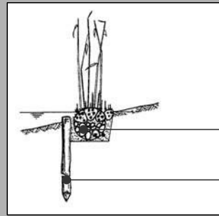
Sezione trasversale
