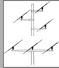
mitigazione attraverso palo rotante
